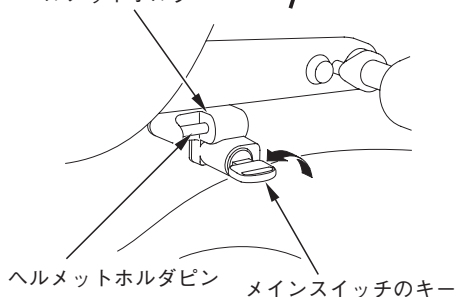
ヘルメットホルダ
